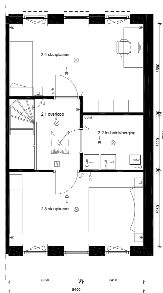
2e verdieping
