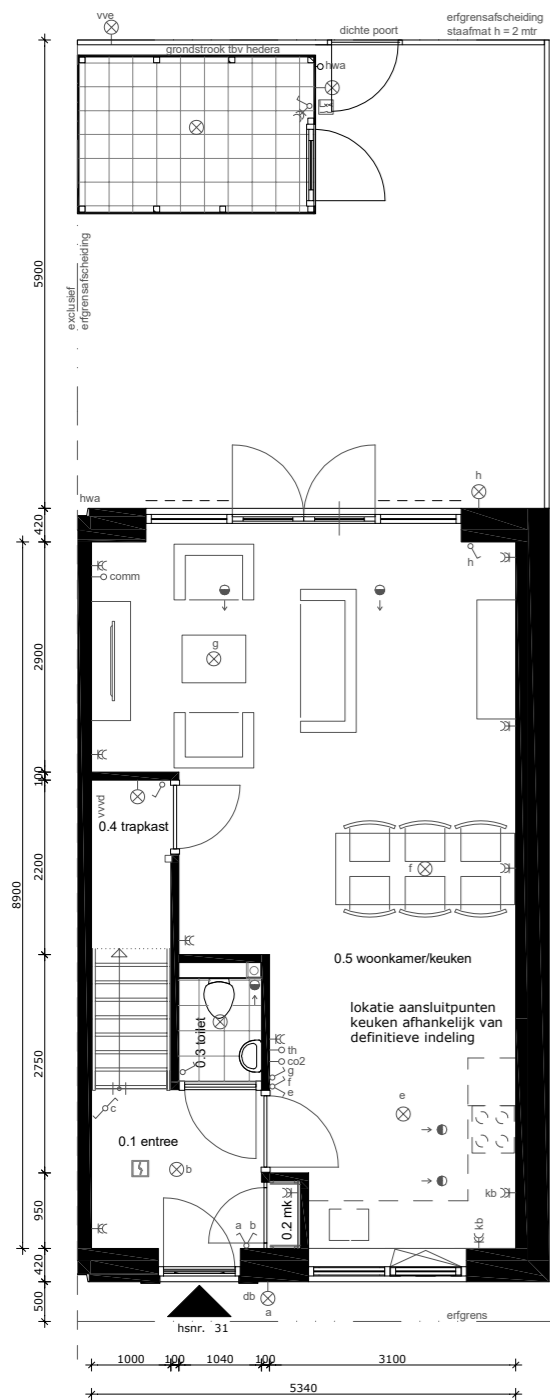
begane grond
